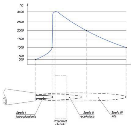
PŁOMIEŃ ACETYLENOWO-TLENOWY
